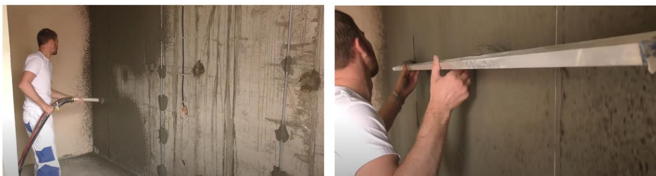
Рис. 25. Схема нанесения обрызга на поверхность и разравнивание правилами образовавшихся наплывов
